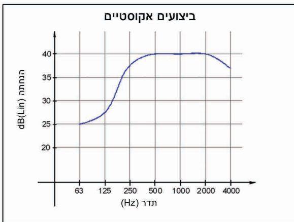
עקומת הנחתה טיפוסית
