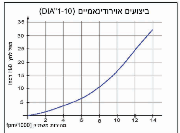
עקומת התנגדות/ מהירות ב-400°C
