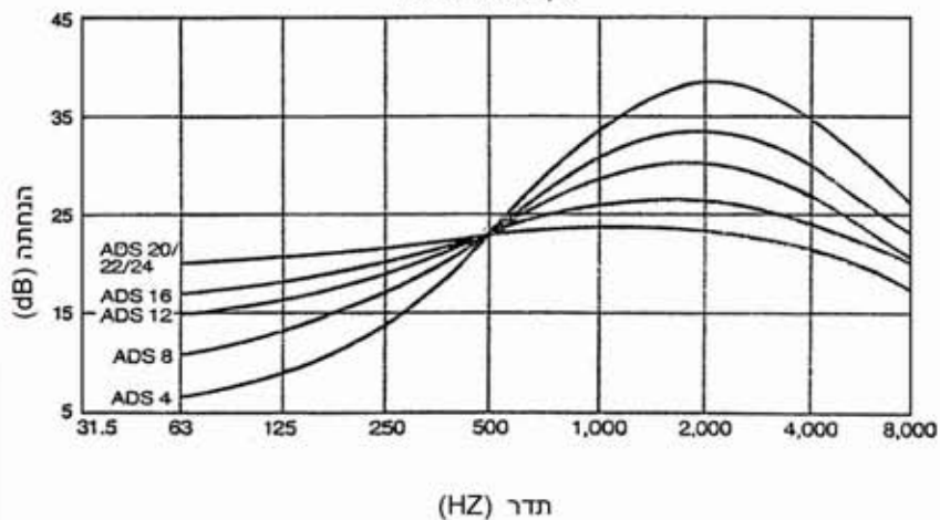
עקומת הנחתה
